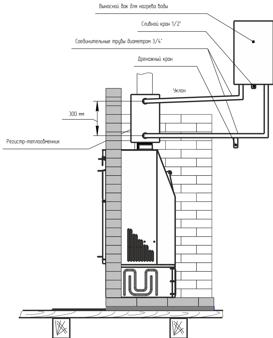
Рис.2 Схема установки дополнительного оборудования
