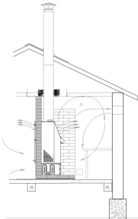
Рис.5 Схема движения воздуха
