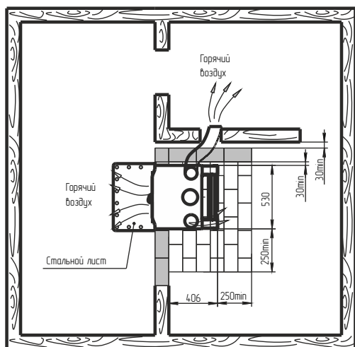
Рис.4 Схема установки камина с воздуховодами
