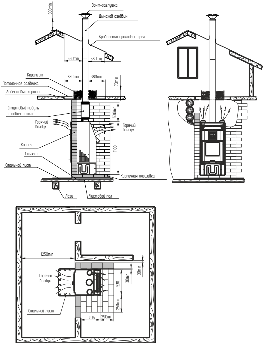
Рис.3 Схема установки камина без воздуховодов
